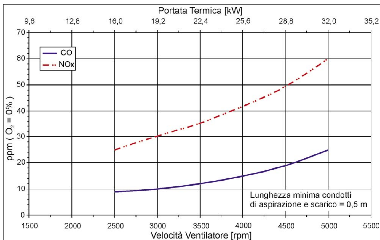
Grafico 7: CURVE CO E NOx (GPL)
