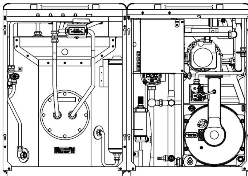
Gruppo termico NB con bollitore affiancato
