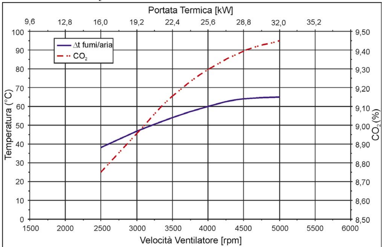
Grafico 8: CURVE CO_2
