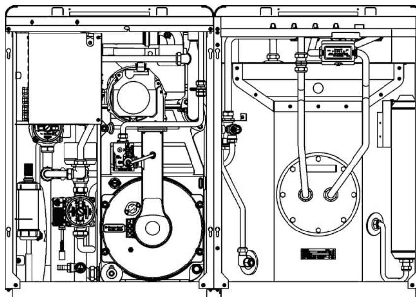
Gruppo termico NB B.T. con bollitore affiancato
