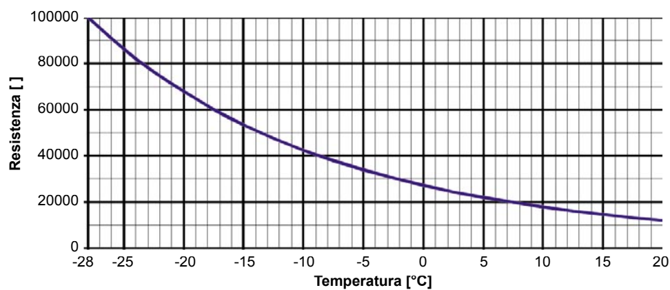
Grafico 13. Valore di resistenza della sonda esterna in funzione della temperatura
