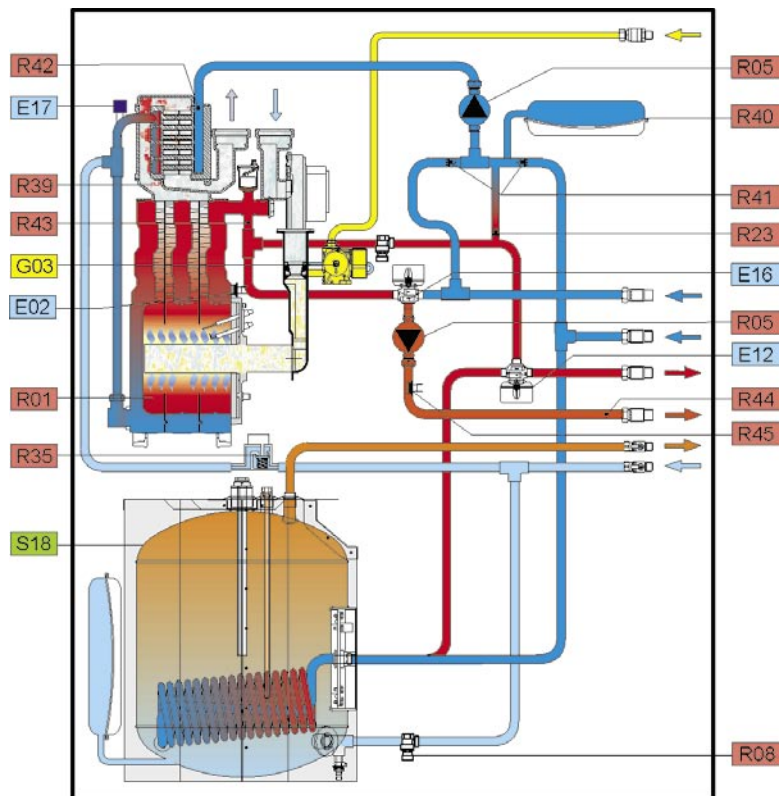
SCHEMA FUNZIONALE NB B.T.
