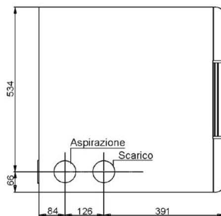
Vista dall'alto
