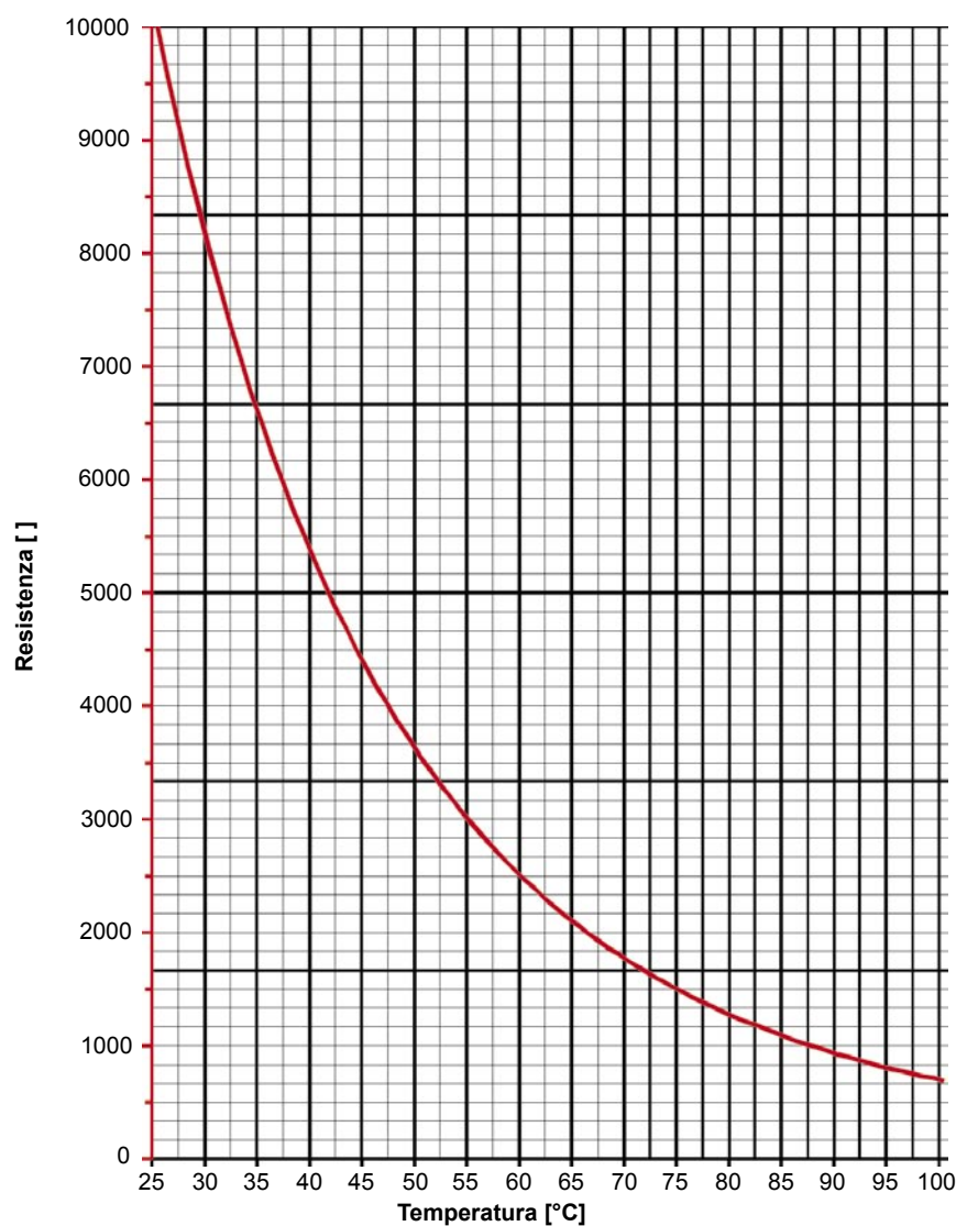
Grafico 13. Valore di resistenza della sonda esterna in funzione della temperatura
