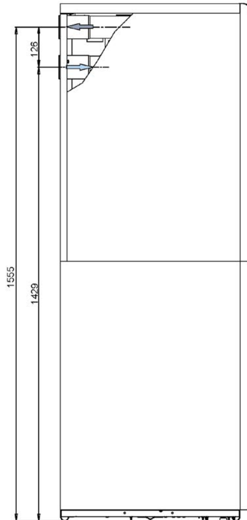
Vista laterale
