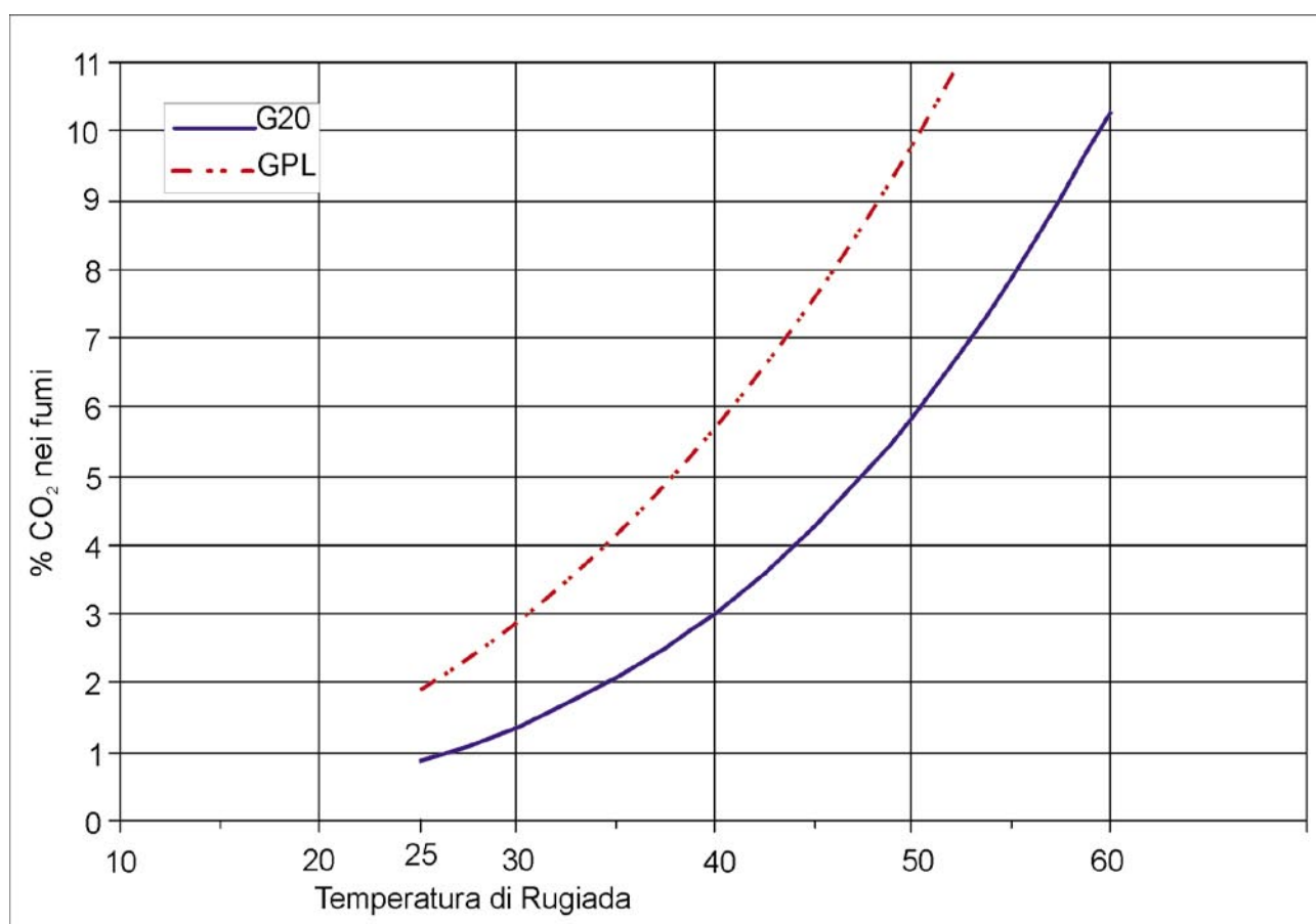
Grafico 11: TEMPERATURA DI RUGIADA
