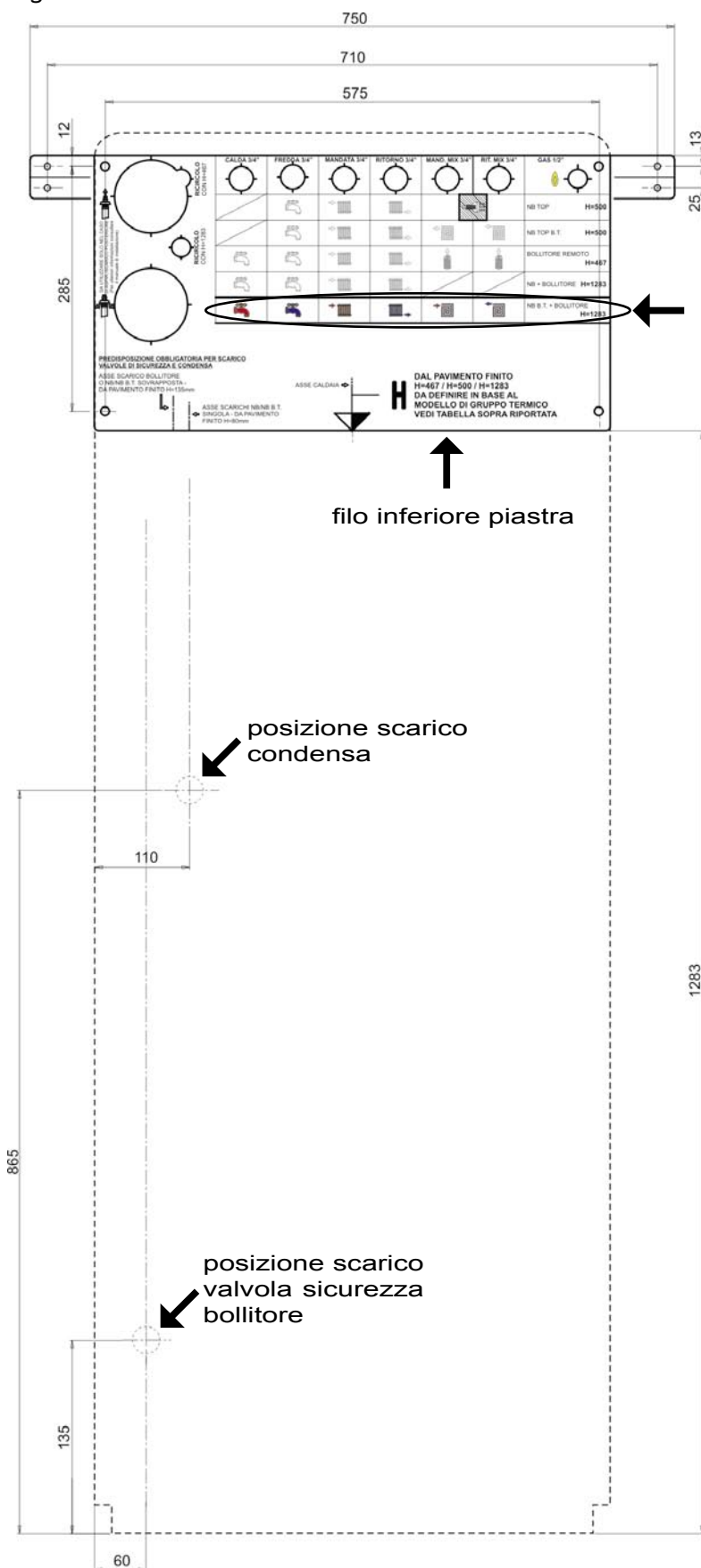
Figura 25 INSTALLAZIONE DEL GRUPPO TERMICO NB B.T. + BOLLITORE
