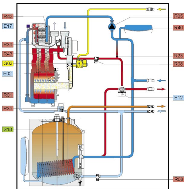
SCHEMA FUNZIONALE NB
