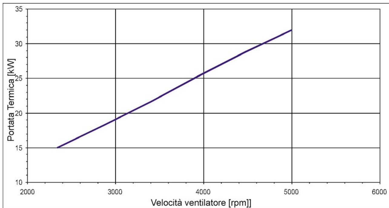
Grafico 10: PORTATA TERMICA
